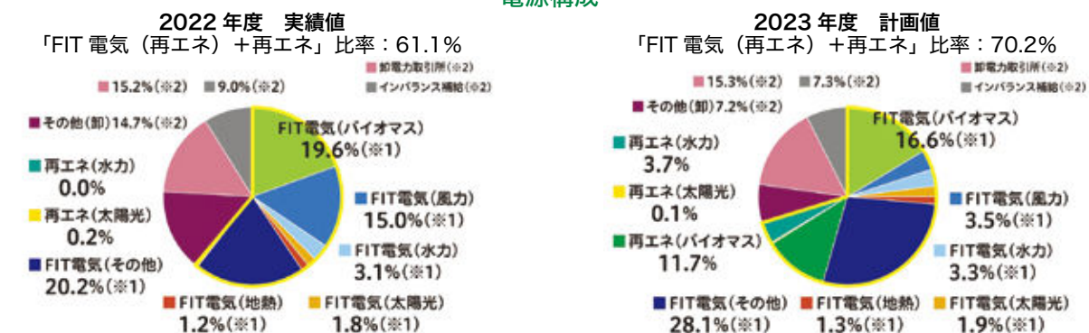
電源構成
